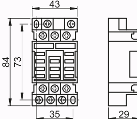
TRACON RSJQX-38FS
