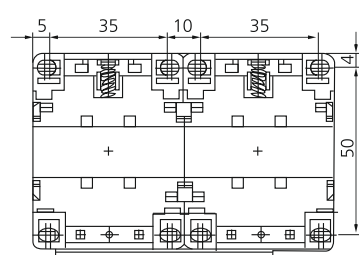
Beépítési méretek / Install size (mm)
