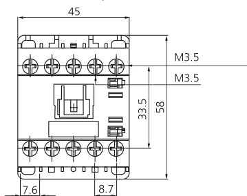
Külső méretek / External dimensions (mm)
