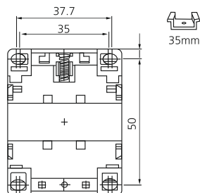
Beépítési méretek / Install size (mm)
