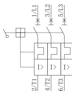
Kapcsolási diagramm / Connection diagramm:
