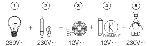
EQ19 (GLS 10÷250W ; LED 0÷100W)
