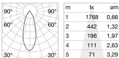
CRI≥90 12W 38° 1000Lm 3000K
