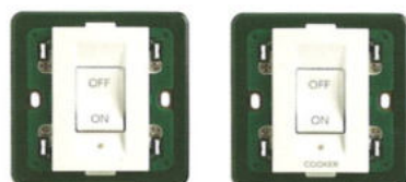
14018 Întrerupător 45 A, ON/OFF. Adâncime: 22,5 mm
