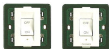
14018 Înterupător 45 A, ON/OFF. Adâncime: 22,5 mm 14018.CK Înterupător 45 A, Cooker. Adâncime: 22,5 mm
