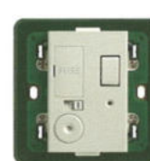
14049.SL 3 Unitate de conexiune 13 A cu întrerupător și siguranță de protecție. Adâncime: 20,4 mm
