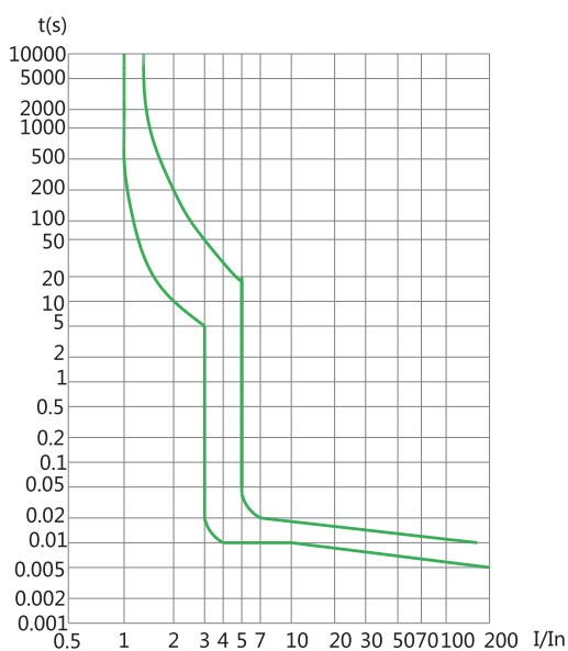
Caracteristica B
