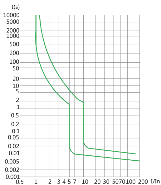
Caracteristica C
