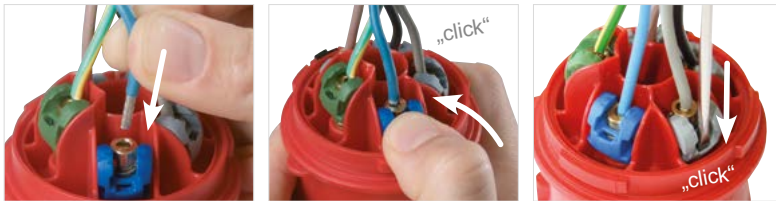
1) Insert wire
