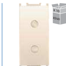
Cod: P-TOP.BG Priză simplă 2P 1M 16AX 250V Bej
