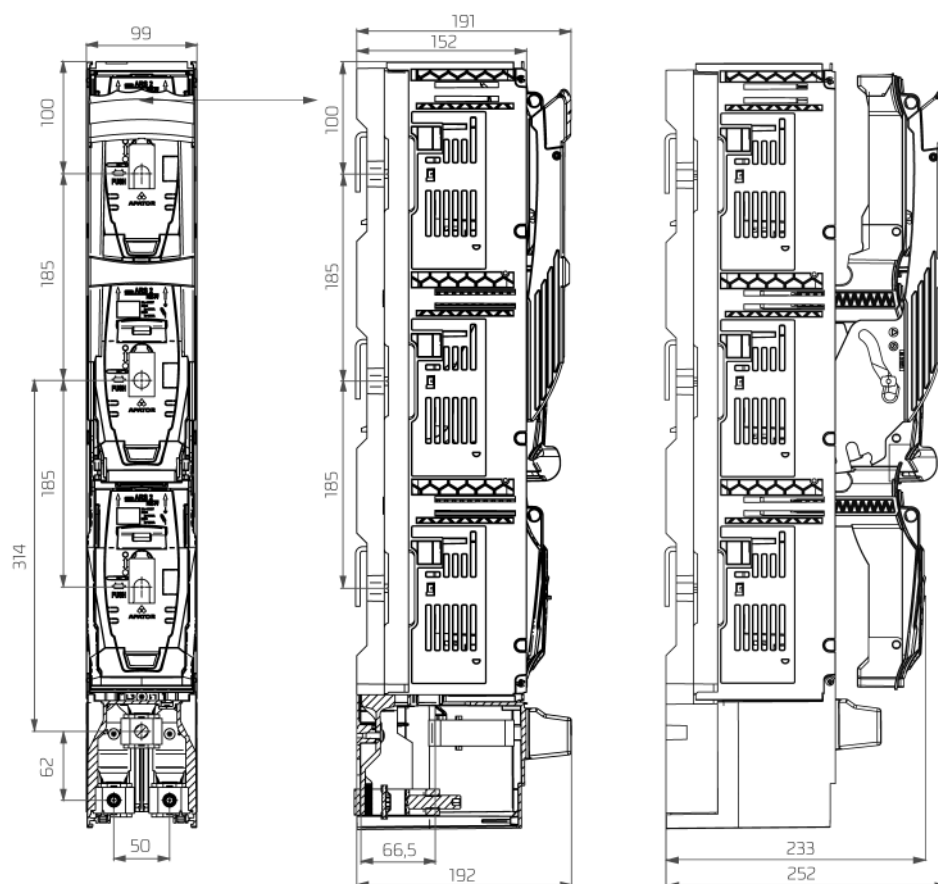
smartARS 2,3 -2V pro-PV
